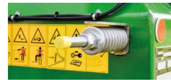
Za pomocą automatycznego napinacza łańcuchów widocznych z ciągnika możliwa jest łatwa regulacja czterech bardzo mocnych łańcuchów przenośnika podłogowego. Dzięki temu uzyskuje się wysoki stopień bezpieczeństwa i jakości działania.
