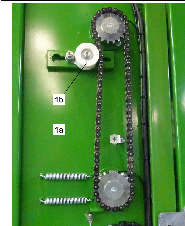
Bild 61: Dosiereinrichtung – Antrieb links
