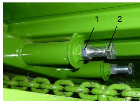
Bild: Spannvorrichtung
