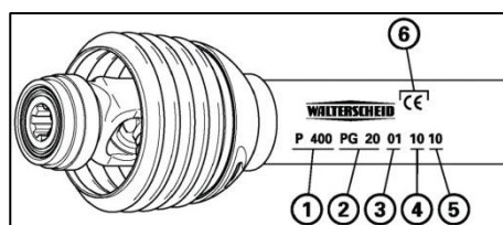
Bild: Gelenkwellen Kennzeichnung
