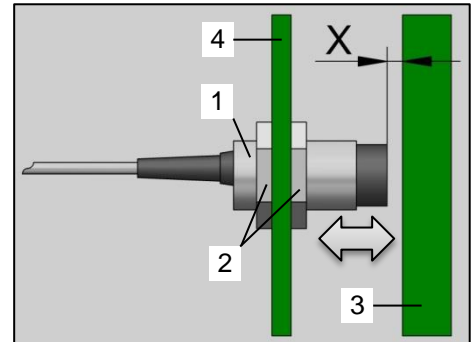
Bild 47: Öffner & Schließer
