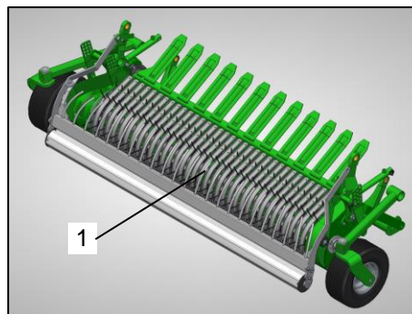
Bild 12: Pick-Up
