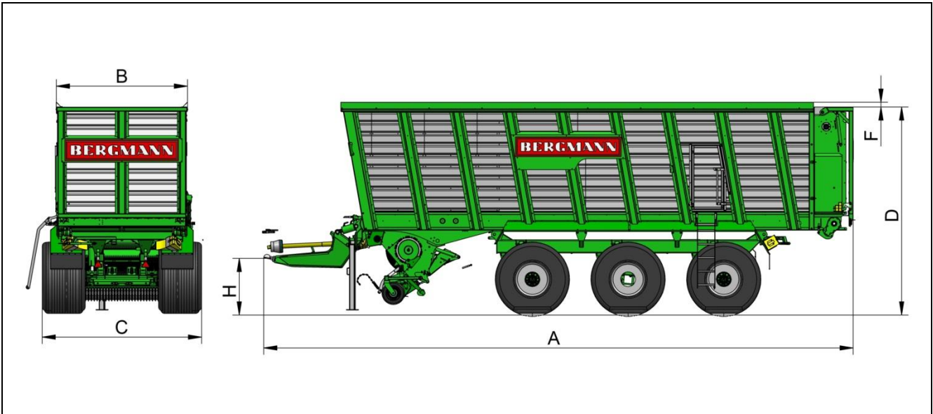
Bild 6: Abmessungen
