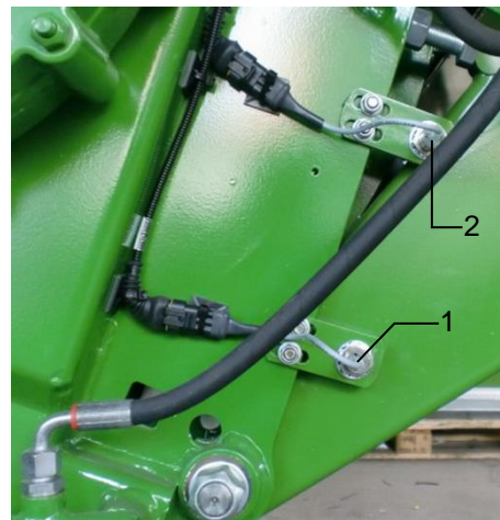
Bild: Schneidwerk
