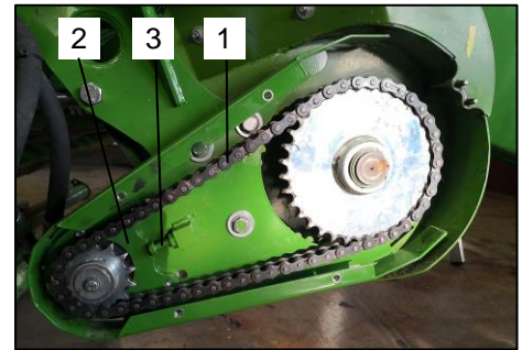
Bild 59: Pick-Up Antrieb
