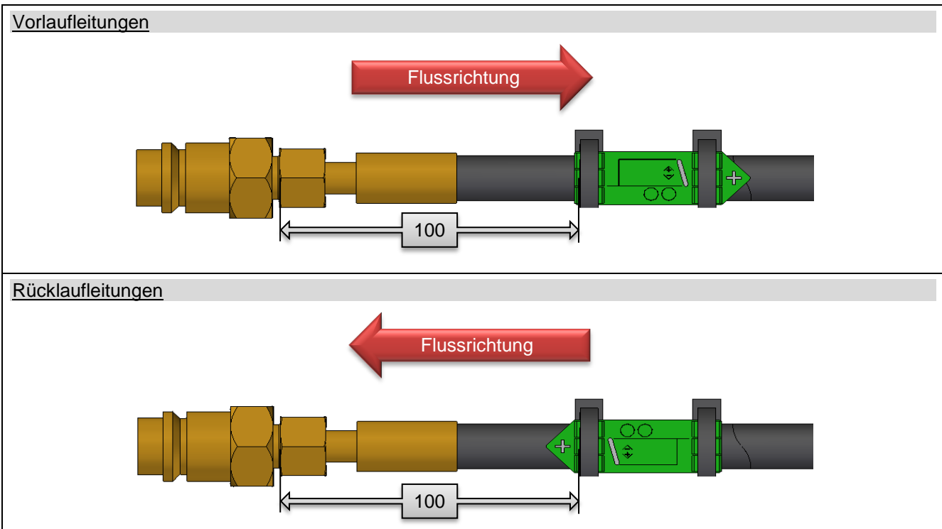
Bild 53: Position der Kennzeichnungen
