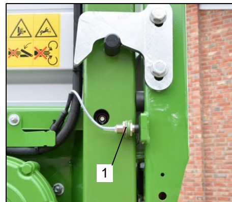
Bild 46: Heckklappen Sensor
