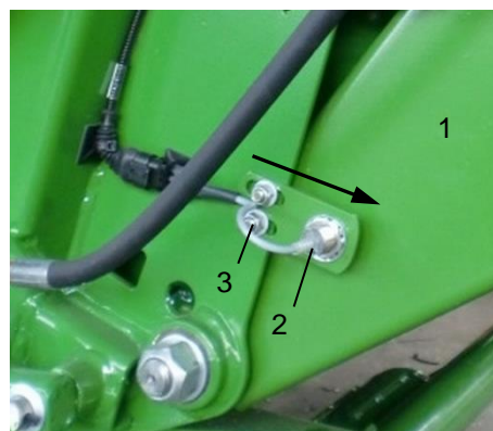
Bild: Sensor unten
