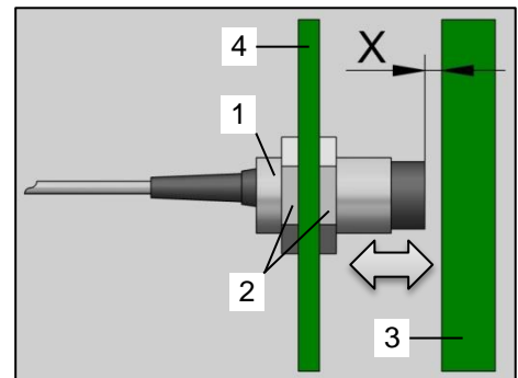
Bild 42: Öffner & Schließer
