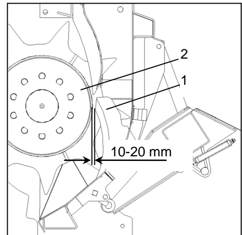
Bild: Messereinstellung
