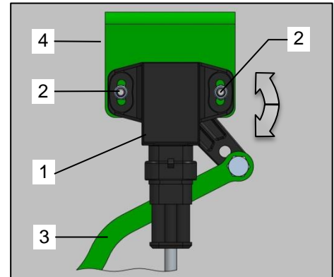
Bild 11: Winkel-Sensor
